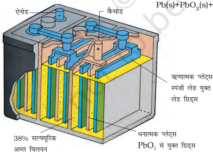
चित्र 2.10—लेड संचायक सेल
